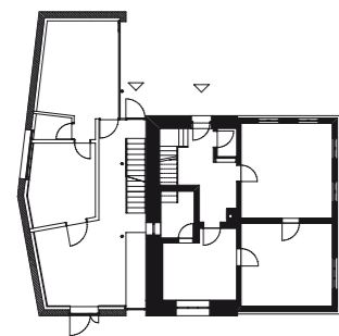
EG +-0.00
