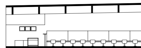
LÄNGSSCHNITT 1
